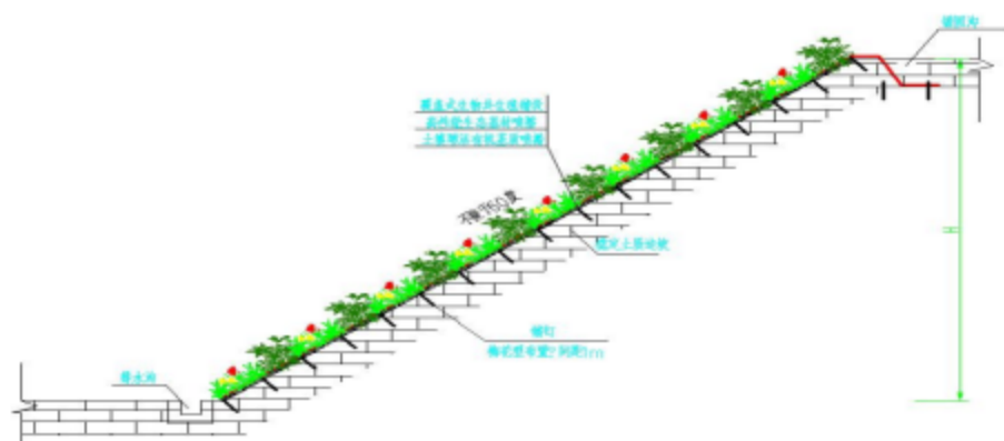
图 3 护坡结构图
