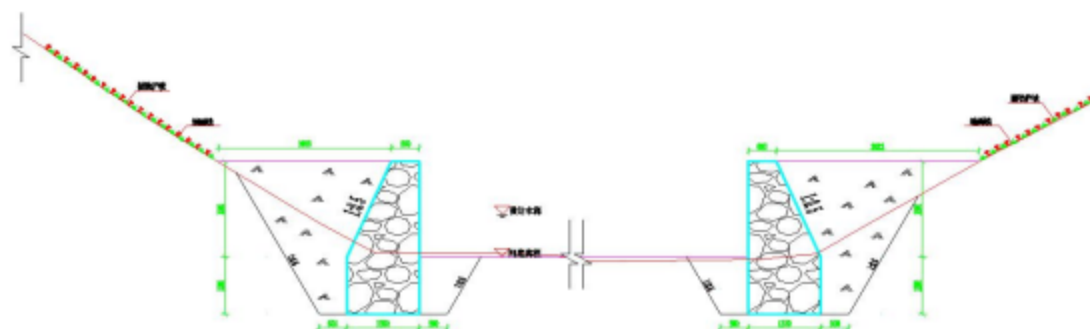
图2 浆砌石式护岸横断面结构图
