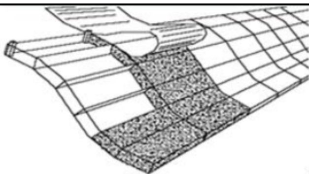
图 6 格宾网垫铺设示意图
