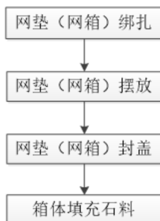
图 4 格宾网垫（网箱）施工工艺流程图
